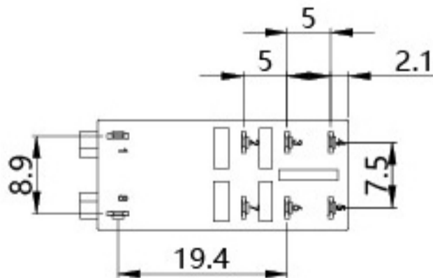
安装尺寸
