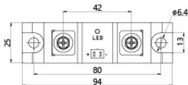
安装尺寸
