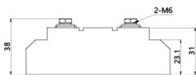
尺寸图
