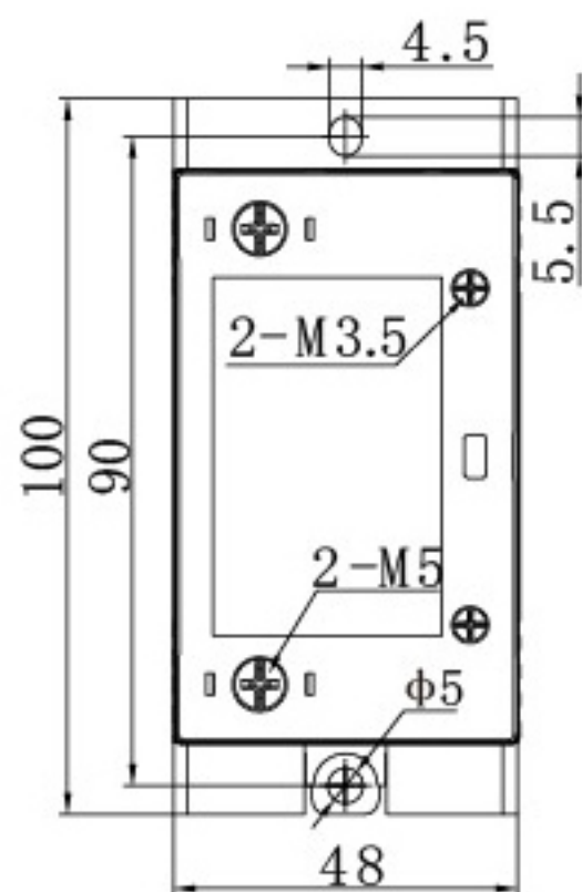
安装尺寸
