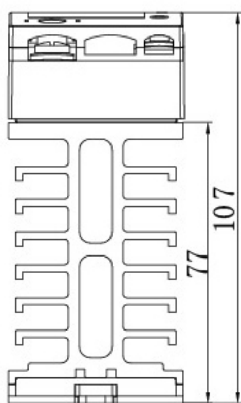
尺寸图
