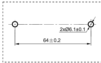
安装孔尺寸
