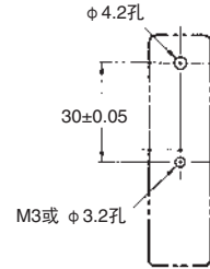
安装孔 (表面连接)
