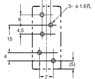
安装孔
