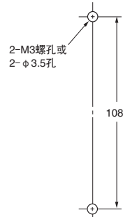
安装孔加工尺寸
