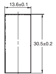
面板开孔
