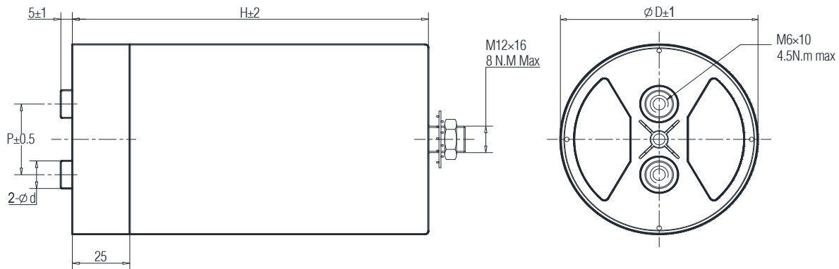
安装孔距与安装螺口外径尺寸 (底部安装螺杆 M12×16, 最大安装扭力 8.0 N.m)
